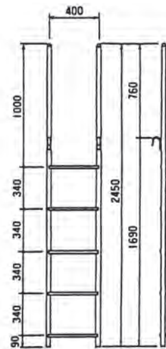
[最上段用] NT-240K (踏面：角型) 12.1kg
