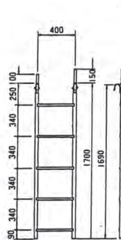
[中・下段用] NT-170K (踏面：角型) 9.9kg
